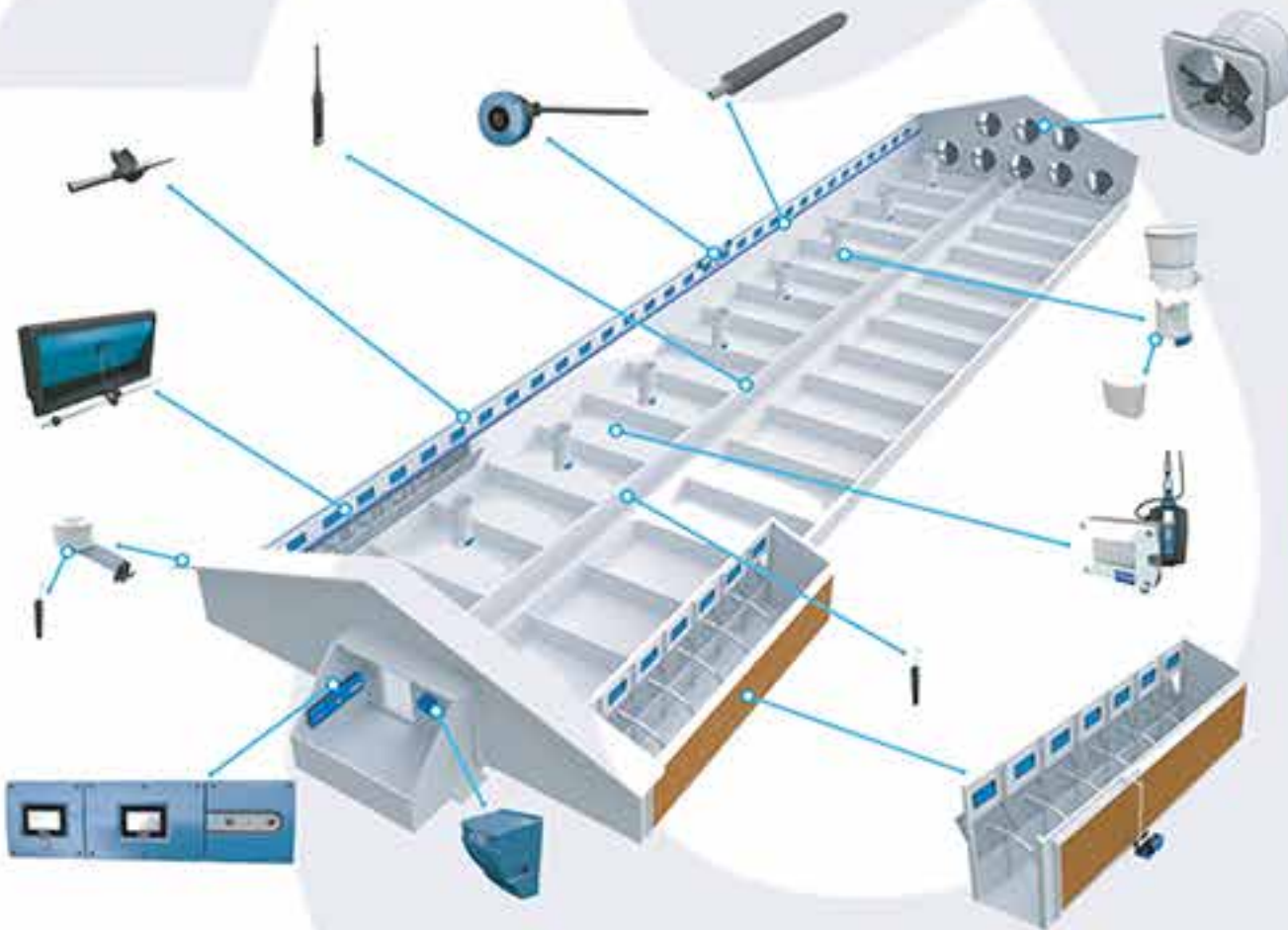
Sistema LPV con entradas laterales.
